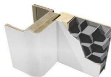
חתך משקוף מדורג + הלבשה רחבה 9 ס"מ
