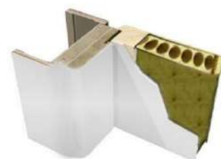
חתך דלת פלקס + משקוף והלבשות עץ
